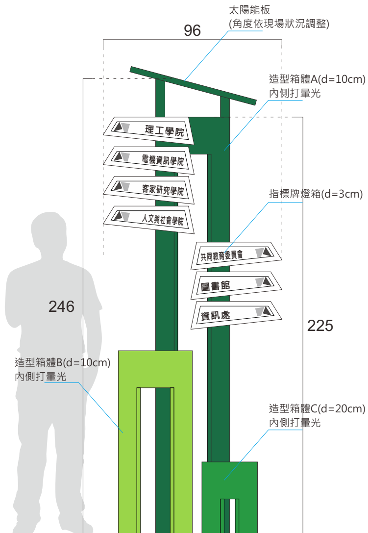
正立面圖
